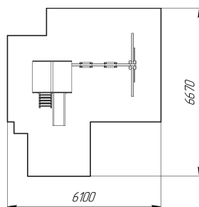
Рис.2 Зона безопасности детской игровой площадки
