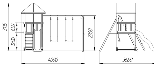
Рис.1 Габаритные размеры детской игровой площадки
