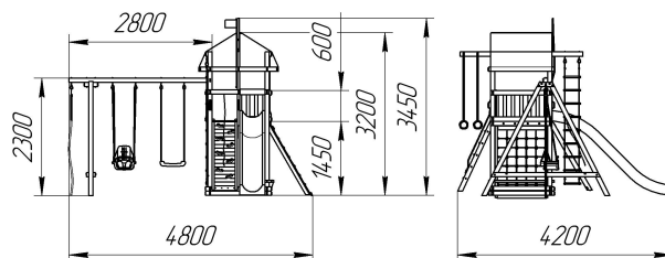
Рис.1 Габаритные размеры детской игровой площадки
