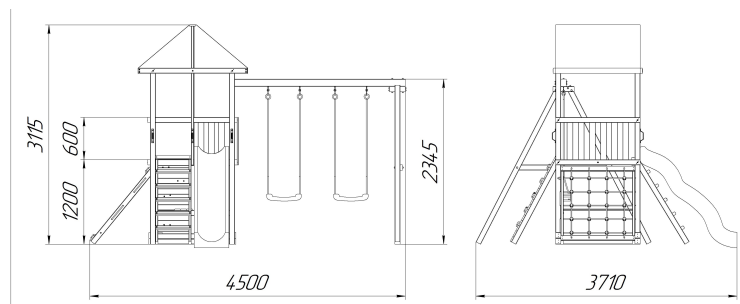
Рис.1 Габаритные размеры детской игровой площадки
