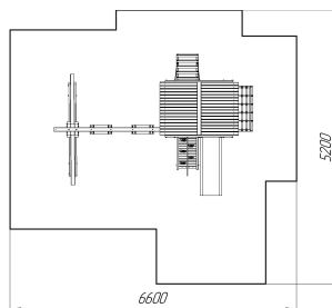
Рис.2 Зона безопасности детской игровой площадки
