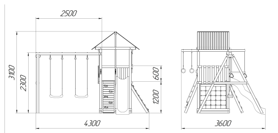
Рис.1 Габаритные размеры детской игровой площадки
